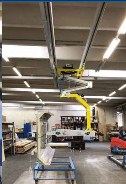
Obračalnik z vodenjem bremena Wendegerät mit Lastführung
