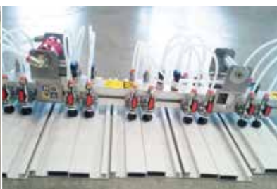
Ročna vakuumska traverza
